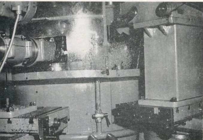
Vue d'une des machines transfert.
