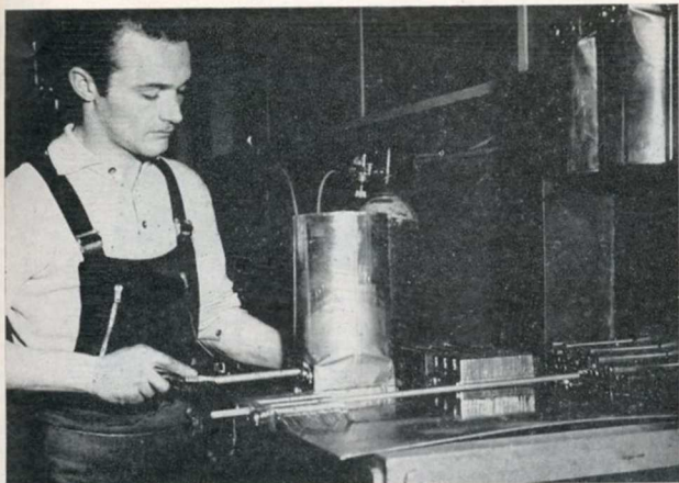
Montage des tubes et des ailettes dans les corps de chauffe.
